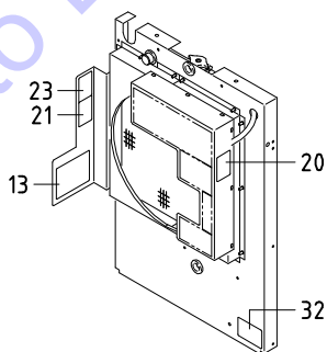
FAN SHROUD
