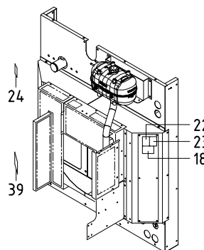
FAN SHROUD
