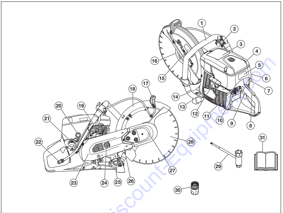
K 770、K 770 OilGuard 動力切割機的構造
