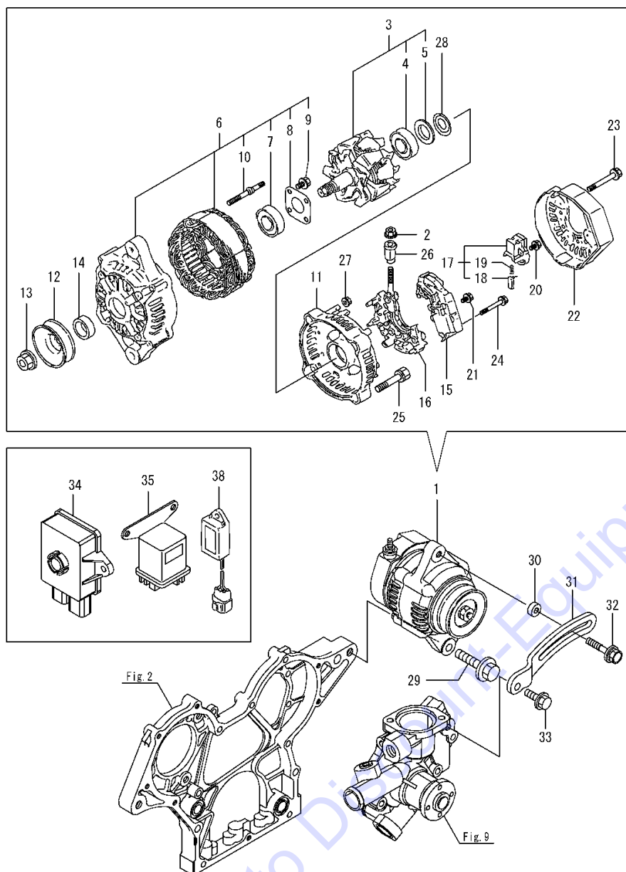
Fig.15. GENERATOR
